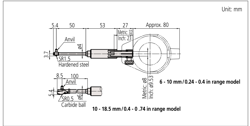
511-209 / 511-214 Anvil
